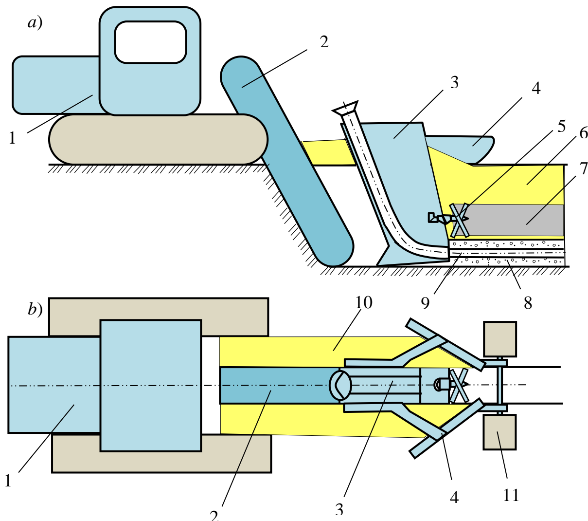
6-rasm. Konstruksiyasi takomillashtirilgan drenaj quruvchi mashina:
