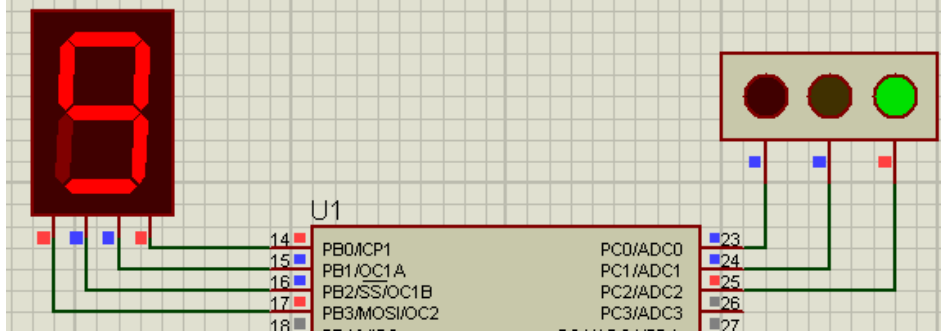
5-rasm. Yashil chiroqni yonish simulyasiyasi.
