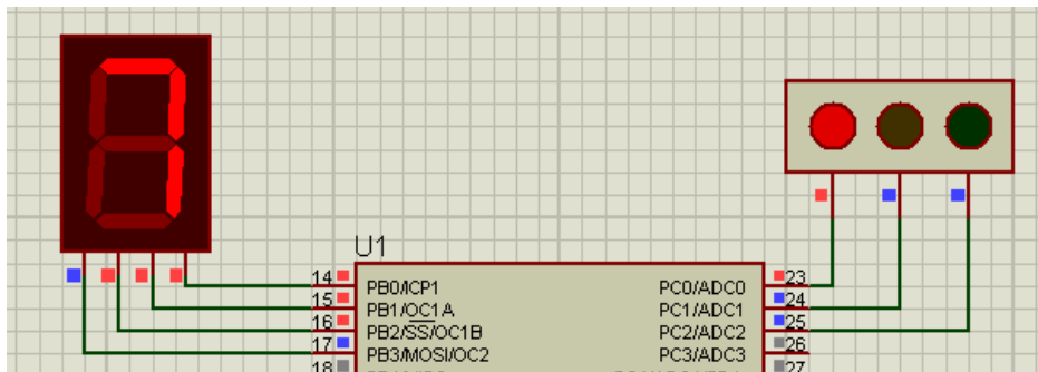
3-rasm. Qizil chiroqni yonish simulyatsiyasi.
