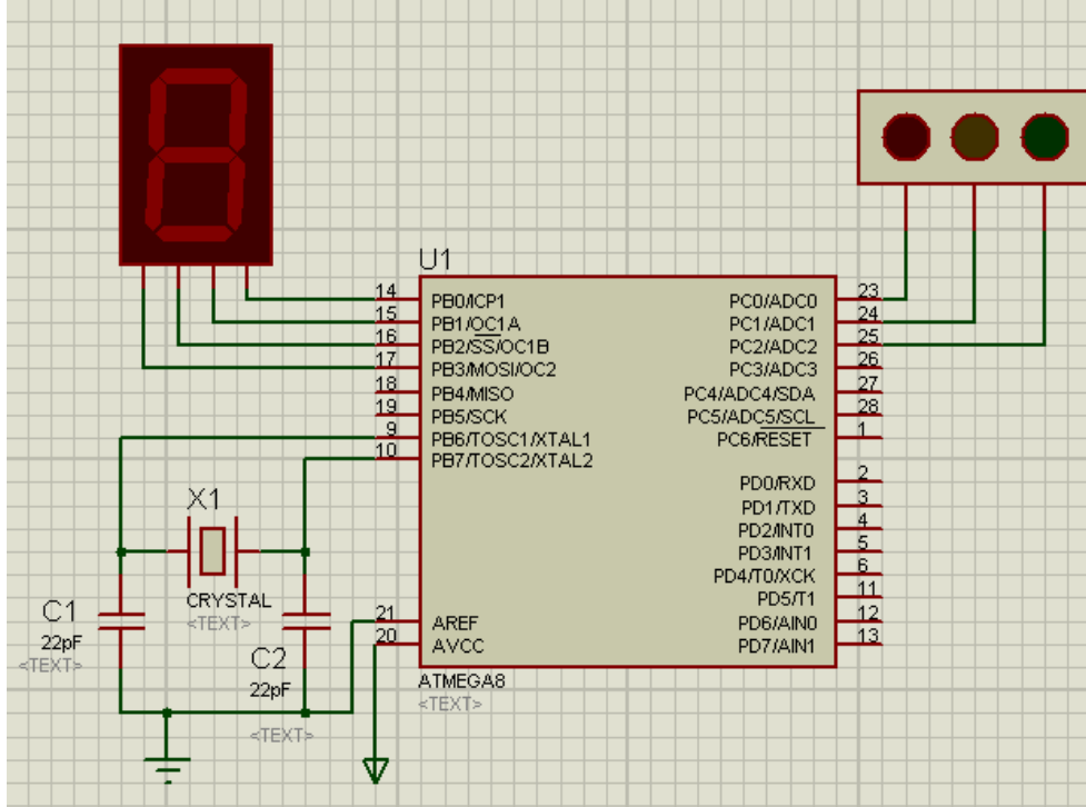
1-rasm. Svetafor tizimini mexatron moduli sxemasi.
