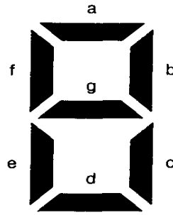
2-rasm. Yetti segmentli display sxemasi.
