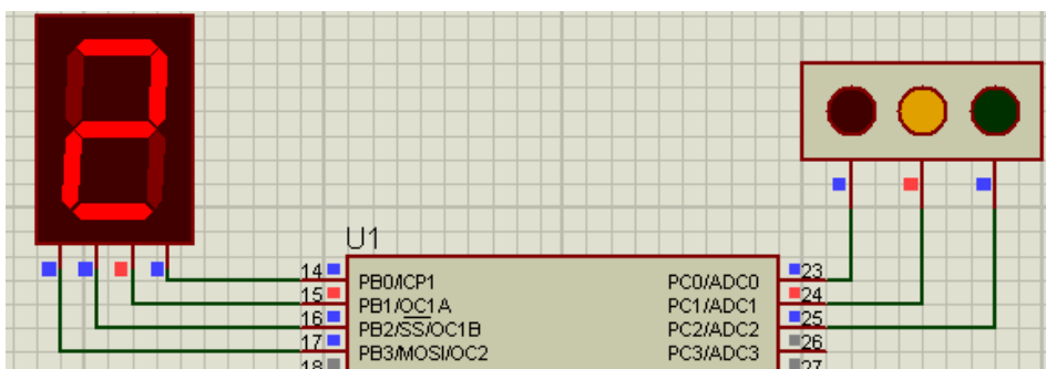
4-rasm. Sariq chiroqni yonish simulyatsiyasi.
