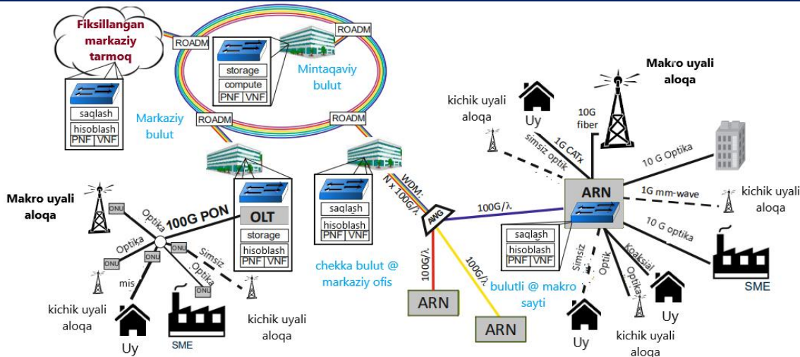
1- rasm. 5G uchun konvergent stasionar mobil tarmoqning jismoniy arxitekturasini.
